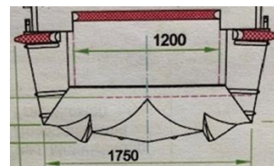
Monorumpf plus Katamaranrumpf
